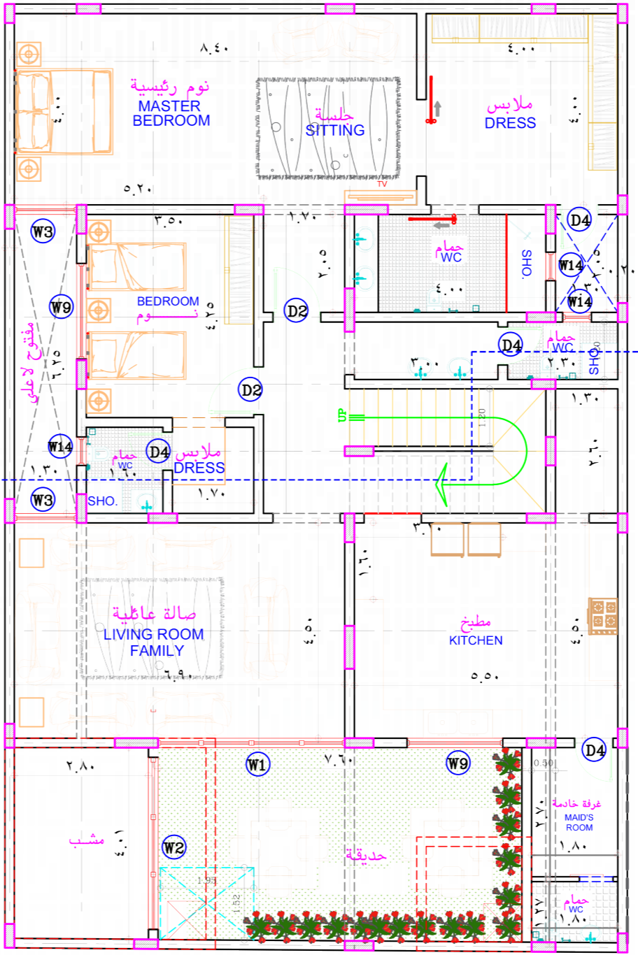
مخطط البدروم
